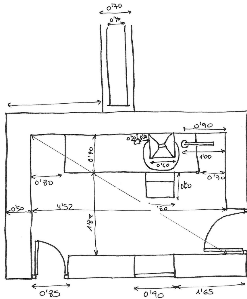
PLANTA
