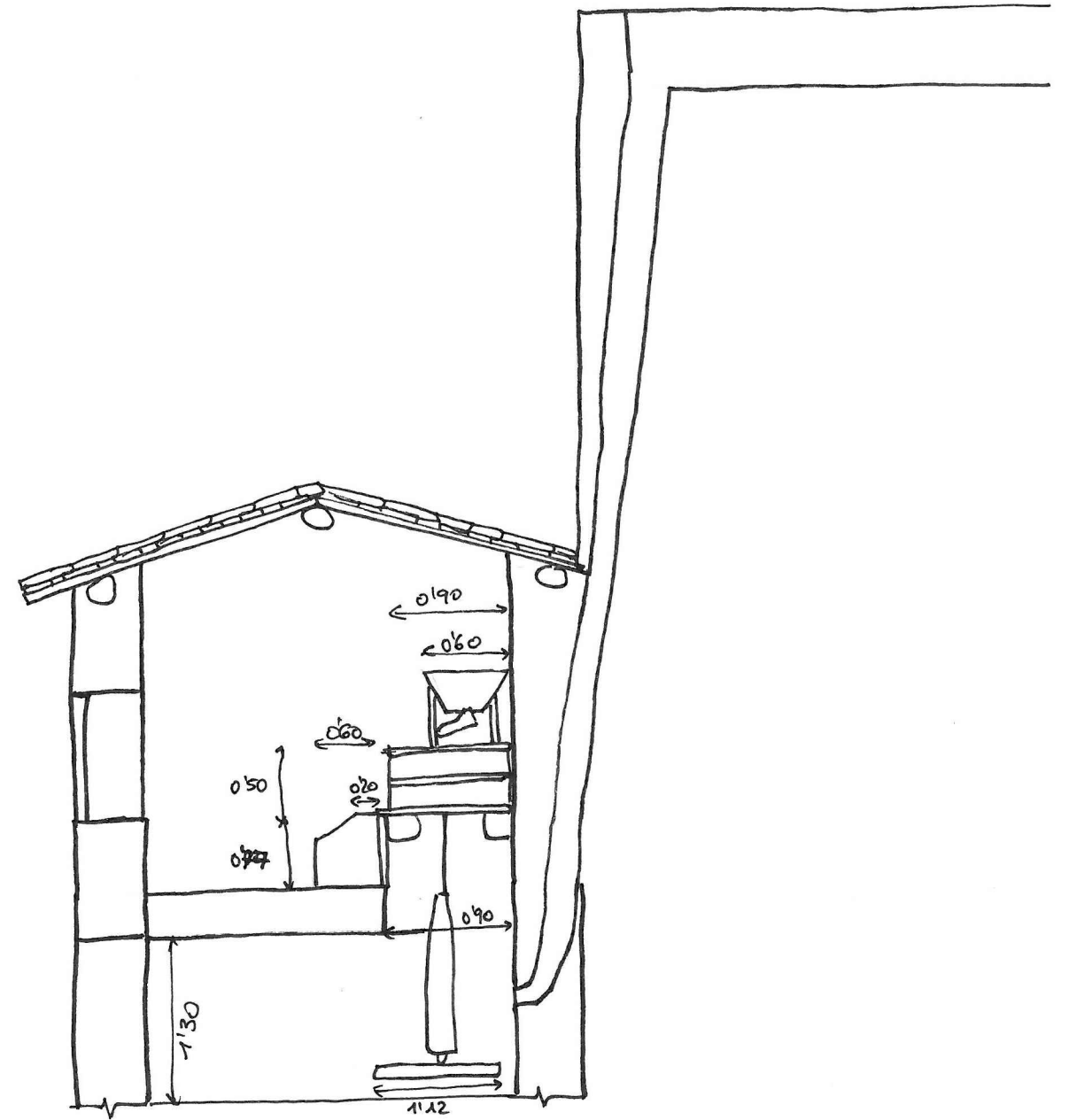
SECCIÓN A-A'
