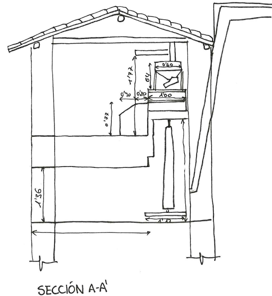
E.A.: PLANTA Y SECCIÓN MOLINO 2
