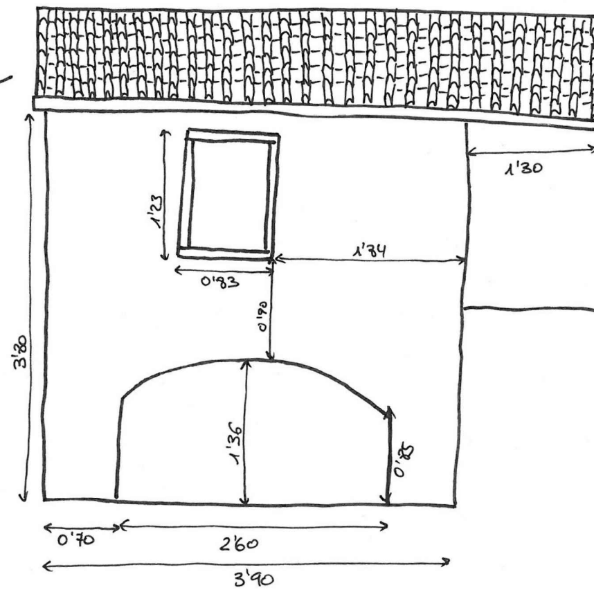
E.A.:ALZADOS MOLINO 2
